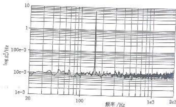
图 A.1 正弦 160 Hz
